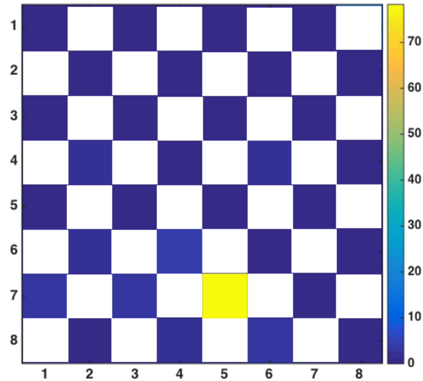
A muon
